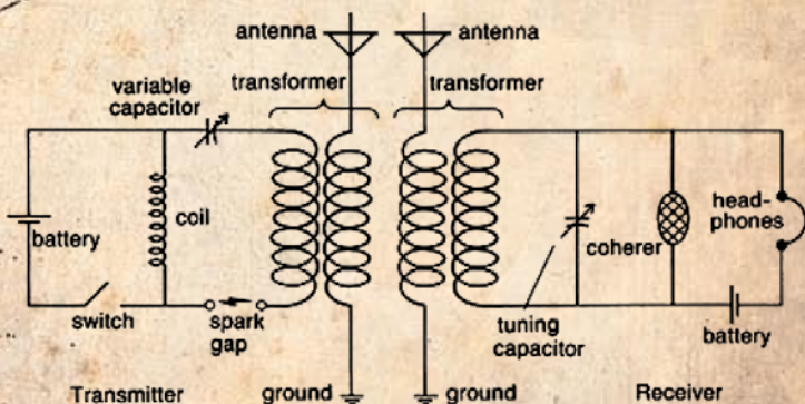
Схемата на първият безжичен предавател на Маркони, изобретен през 1900г.
